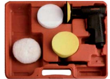
US-1057/1 Disco abrillantador 1/2" bonnet
